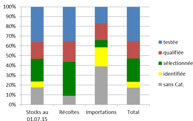
Graphique 9 : Répartition des graines disponibles par catégorie commerciale des essences résineuses en 2015-2016
