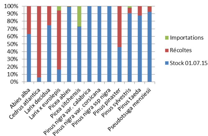
Graphique 8 : Répartition de l’approvisionnement en graines des principales essences résineuses en 2015-2016
