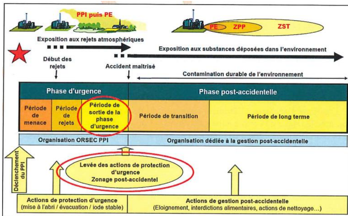
Illustration 1 : phases d'un accident nucléaire majeur (sources : ASN)
