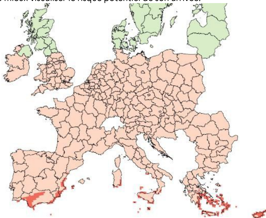
Carte 1 : Aires de distribution potentielles de Spodoptera frugiperda (EFSA, 2019)
