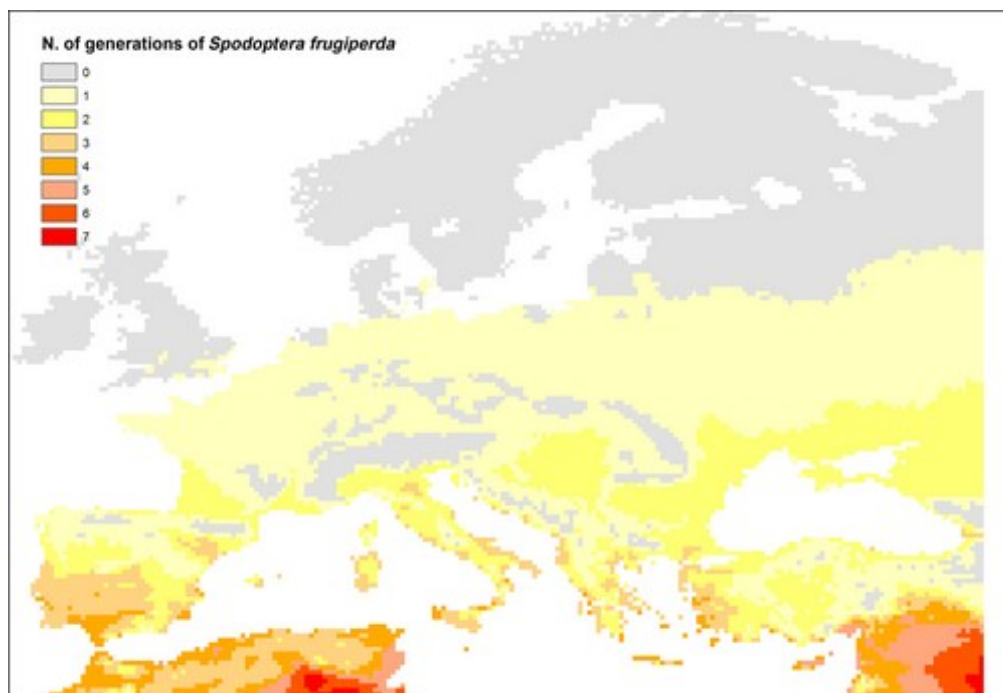
Carte 2 : Nombre de cycles de vie que S. frugiperda peut effectuer sur un an (EFSA, 2019)
