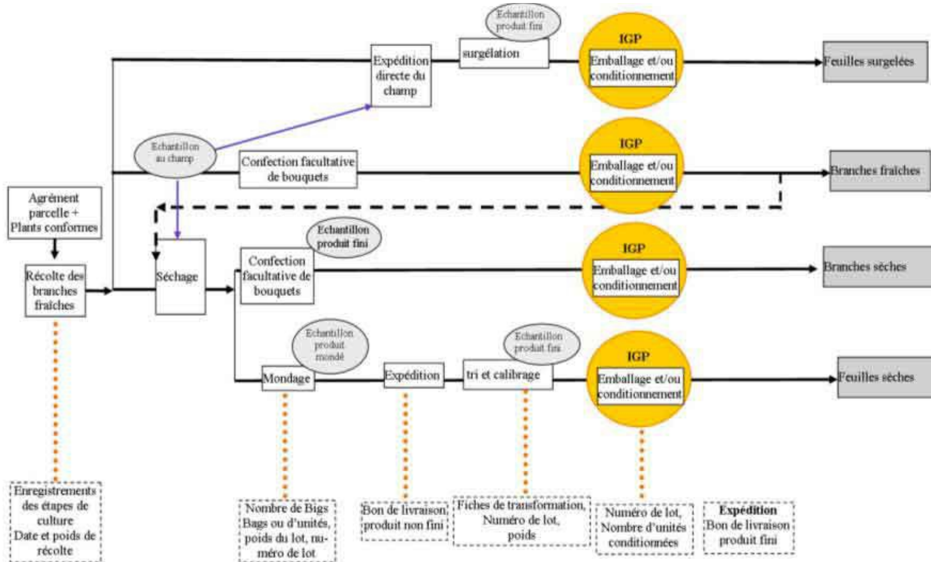
SCHÉMA 1: TRAÇABILITÉ ASCENDANTE ET DESCENDANTE
