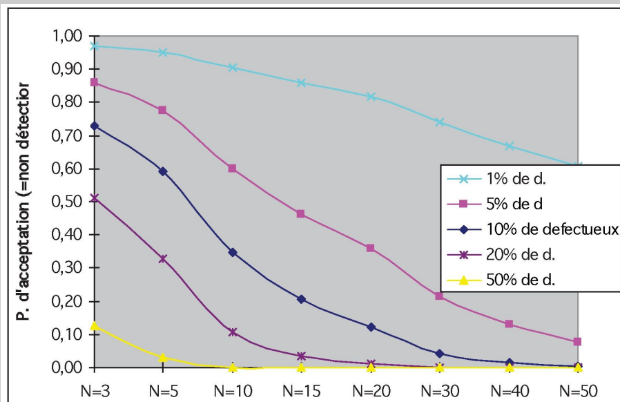
Illustration 2: Incidence de l'effectif d'échantillon sur l'efficacité des plans pour différentes qualités de lots (les plans sont de type c=0 ; les courbes sont établies à partir de calculs selon la loi binomiale) ; extrait de la note de service DGAL/SDSSA/N2008-8009 du 14 janvier 2008
