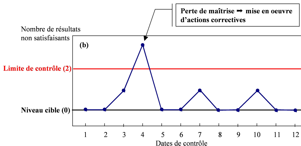
Illustration 4: Exemple de carte de contrôle pour le suivi à long terme des résultats d'analyses microbiologiques (AFSSA, sept 2008) ; le niveau cible et la limite de contrôle doivent être déterminés par l'exploitant en fonction de l'historique des données sur son site.
