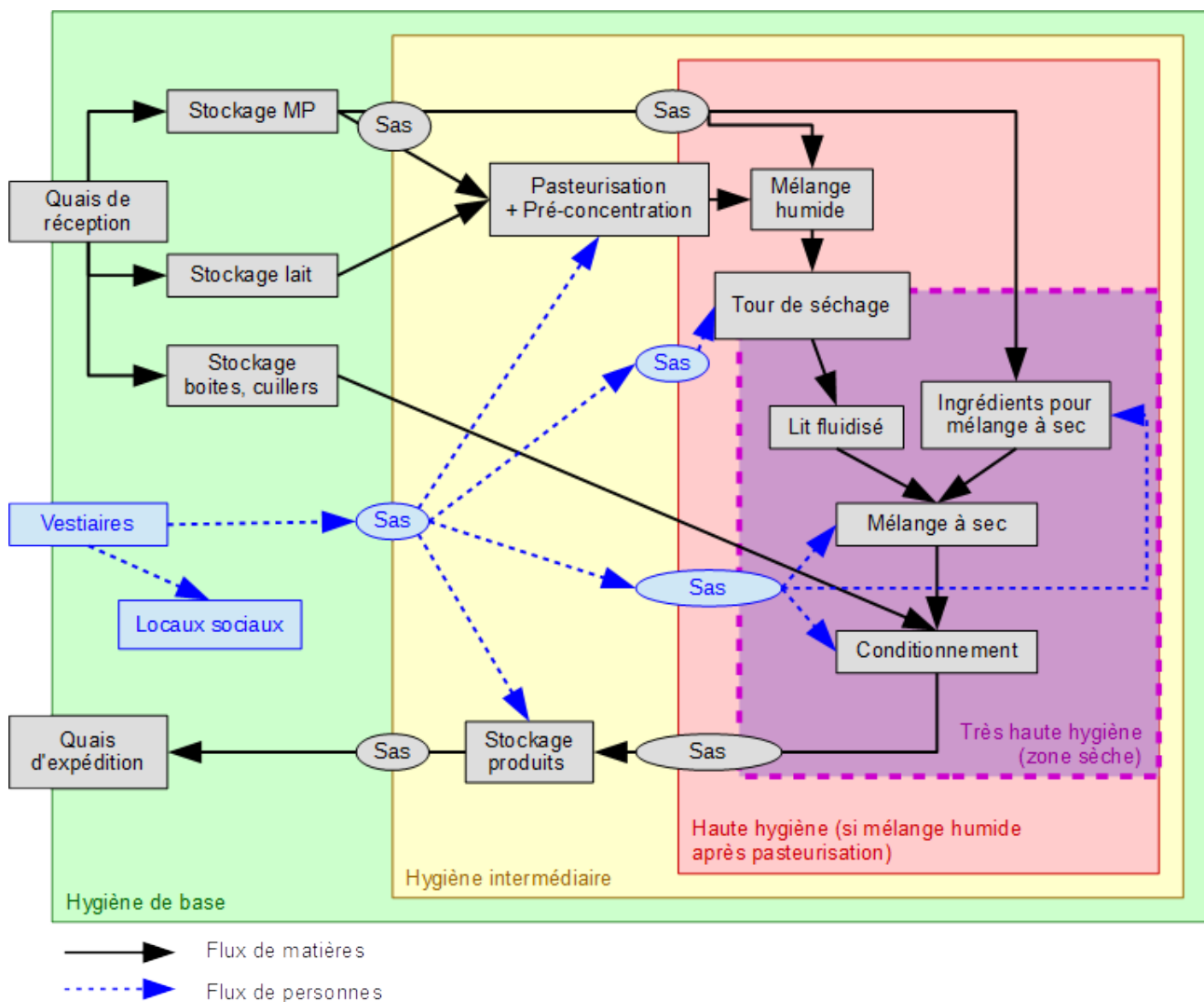
Illustration 1: Schéma de principe de la sectorisation des locaux de fabrication de poudres de lait infantile
